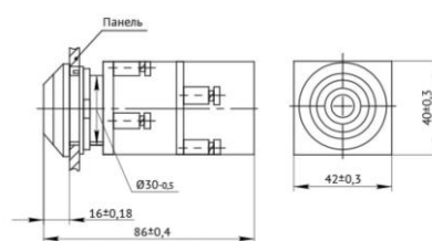
Рисунок 6. Выключатель кнопочной KE-082
