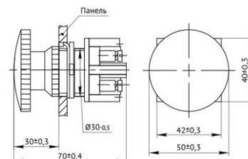
Рисунок 3. Выключатель кнопочной KE-021
