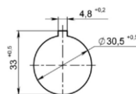
Рисунок 11. Размеры установочного отверстия в панели для установки выключателей кнопочных KE
