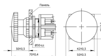
Рисунок 9. Выключатель кнопочной KE-191
