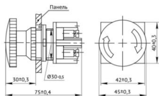
Рисунок 7. Выключатель кнопочной KE-131; KE-141
