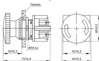
Рисунок 10. Выключатель кнопочной KE-201
