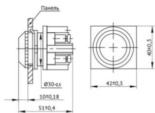
Рисунок 1. Выключатель кнопочной KE-011
