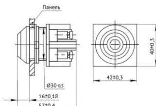
Рисунок 5. Выключатель кнопочной KE-081
